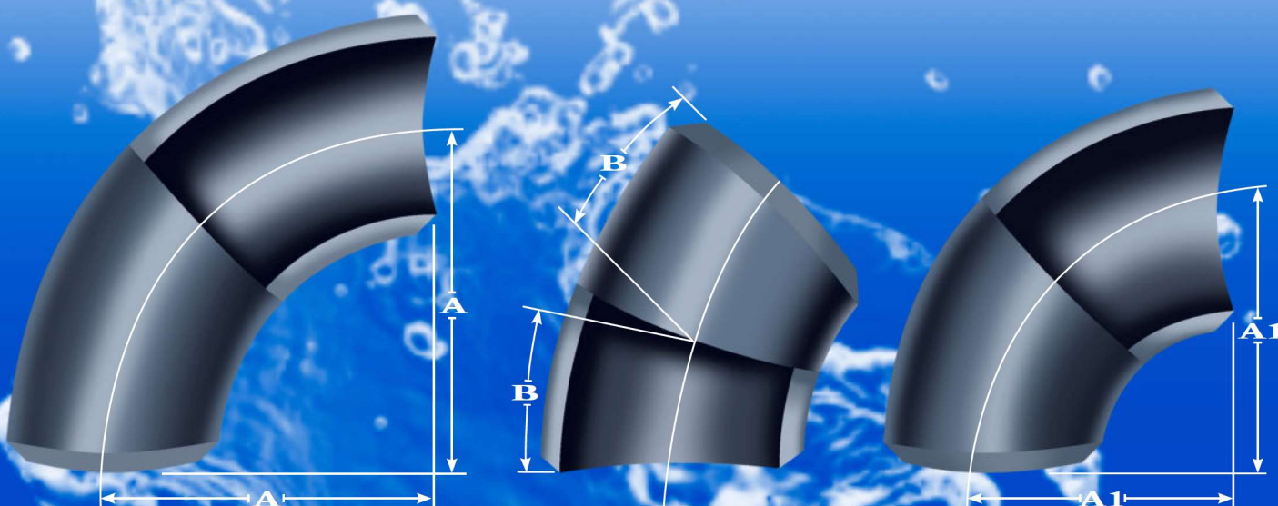
Codo 90° R.L.
